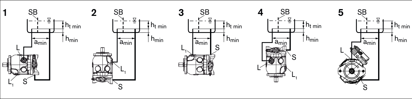
Abb. 7: Untertankeinbau A10VO/A10VSO mit Einbaulage 1–5
