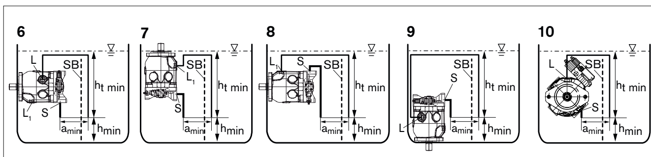
Abb. 8: Tankeinbau A10VO/A10VSO mit Einbaulage 6–10
