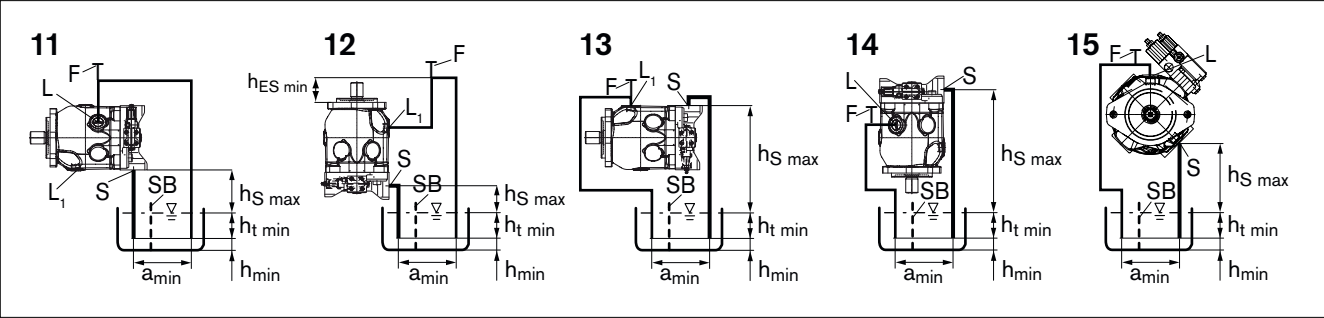
Abb. 9: Übertankeinbau A10VO/A10VSO mit Einbaulage 11–15
