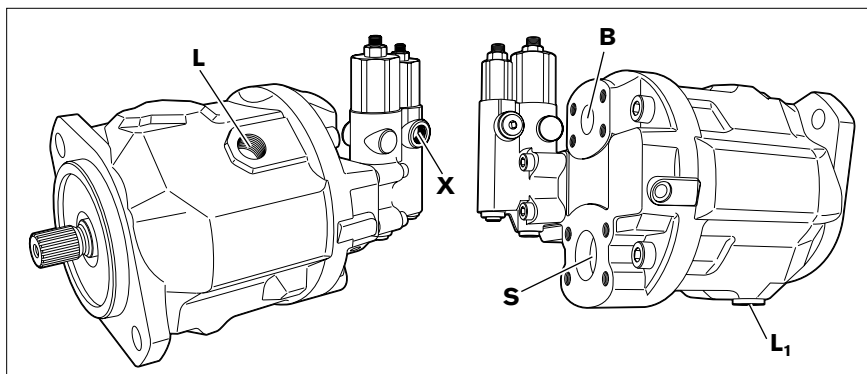
Abb. 12: Anschlussübersicht A10VO Baureihe 31, SAE-Flanschanschlüsse hinten
