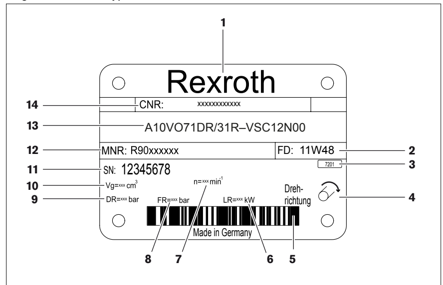
Abb. 3: Typschild A10VSO
