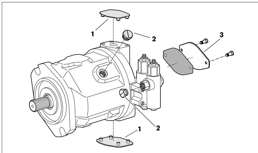
Abb. 11: Transportschutz entfernen
