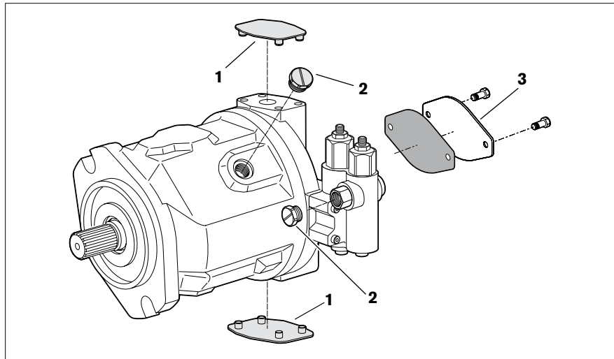
Abb. 1: Axialkolbeneinheit A10VSO
