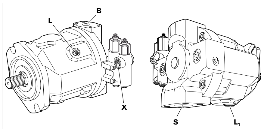
Abb. 13: Anschlussübersicht A10VO/A10VSO Baureihe 31, SAE-Flanschanschlüsse oben, unten gegenüberliegend
